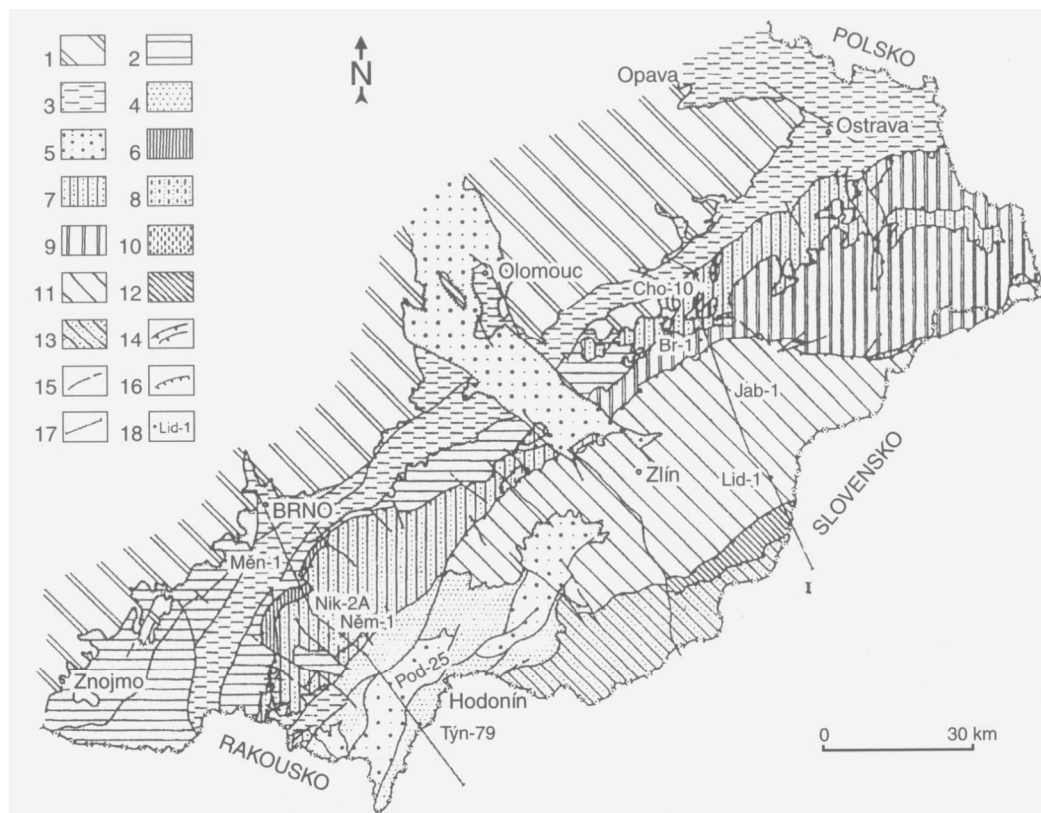
Obr. 6. Regionální geologické dělení Západních Karpat na našem území (podle usnesení České stratigrafické komise 1994, 1995). 1 – Český masiv; 2 – spodní miocén karpatské předhlubně (eggenburg–karpát); 3 – střední miocén (baden); 4 – svrchní miocén (sarmat–pannon); 5 – pliocén; 6 – pouzdřanská jednotka; 7 – ždánická a podslezská j.; 8 – zdounecká j.; 9 – slezská j.; 10 – předmagurská j.; 11 – račanská j. magurské skupiny příkrovů; 12 – bystrická j. magurské skupiny příkrovů; 13 – bělokarpatská j. magurské skupiny příkrovů; 14 – příkrový a přesmykový; 15 – zlomy; 16 – okraj transgrese; 17 – linie geologických řezů; 18 – vrty.
